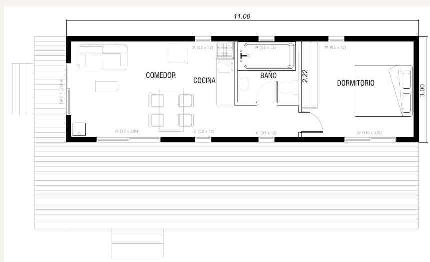
PLANTA ARQUITECTÓNICA · DECK EXTERIOR
